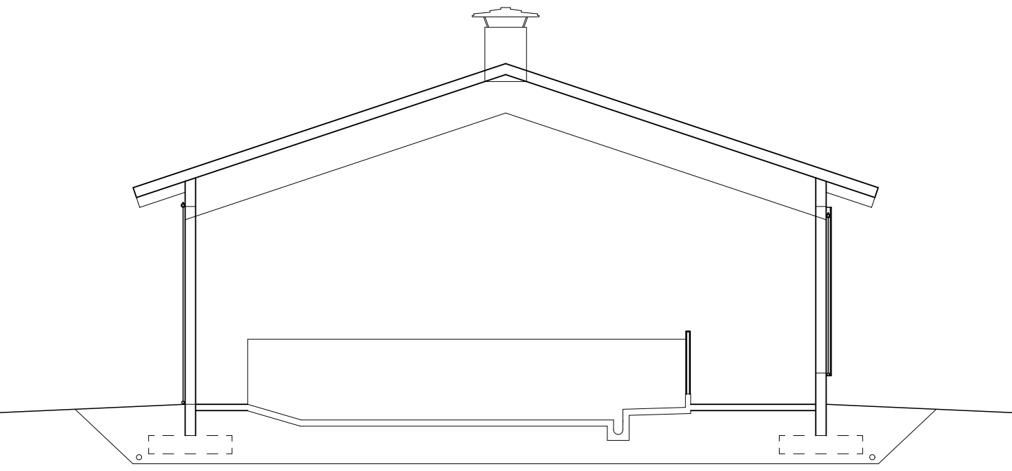
LEIKKAUS B-B
