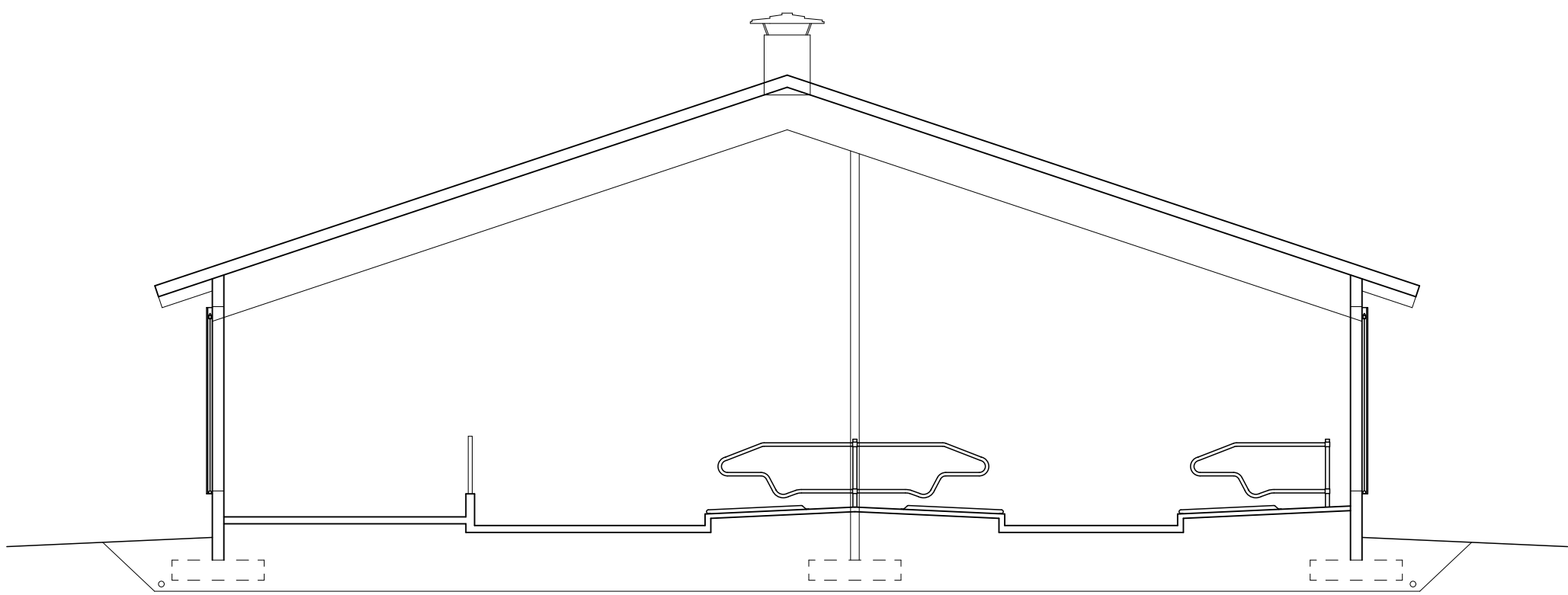
LEIKKAUS A-A
